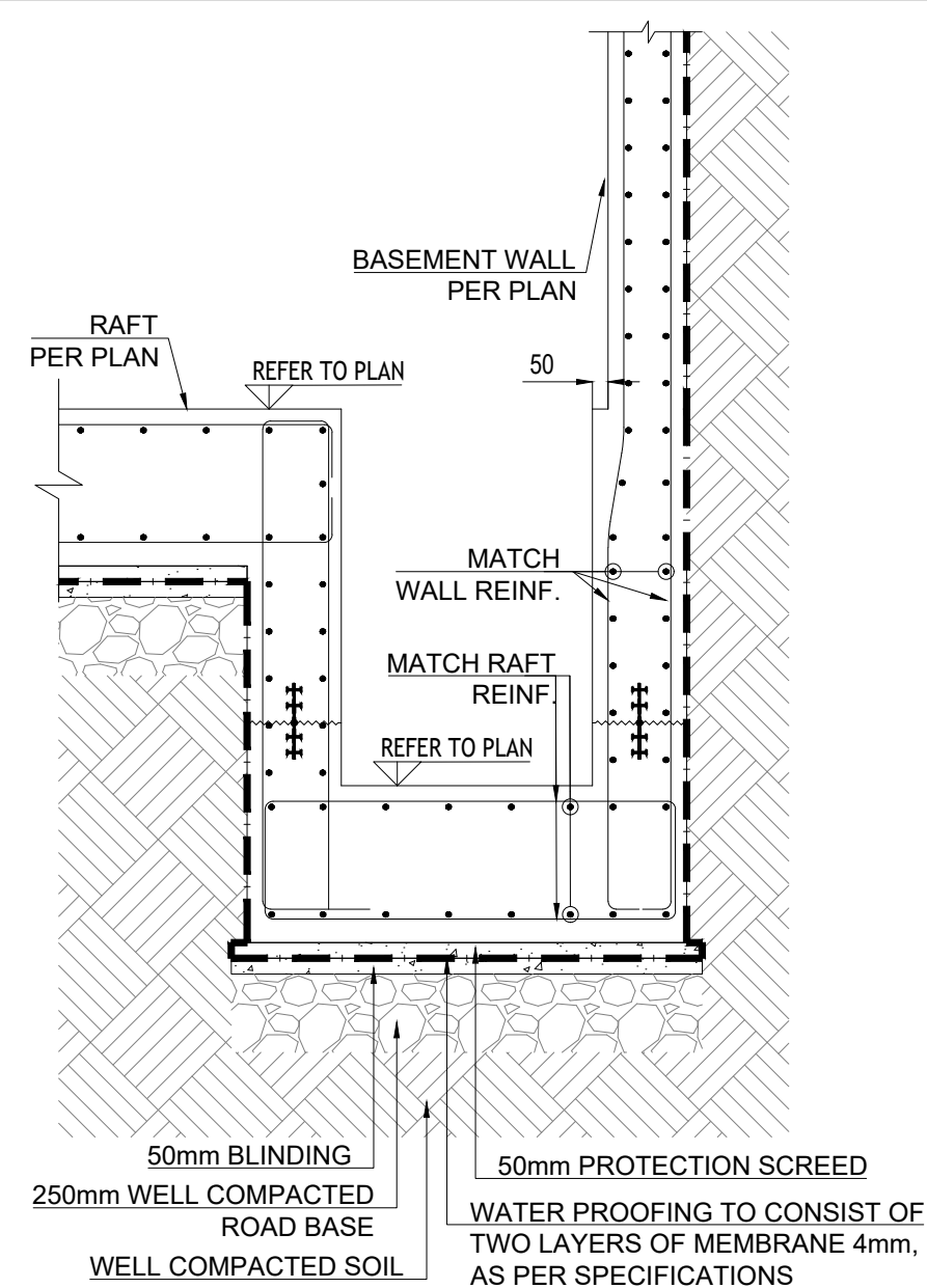
B4 S-100 SUMP PIT SECTION SCALE: 1:25
